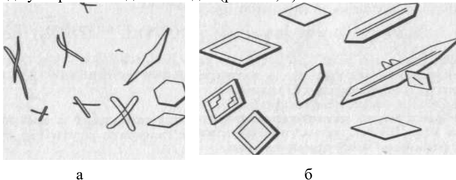
Рис. 6. Кристаллы сульфата свинца (а) и сульфата серебра (б)
